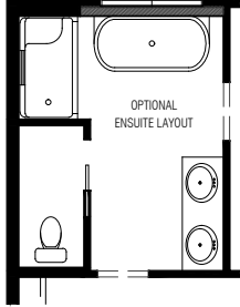
ENSUITE #1 LAYOUT
